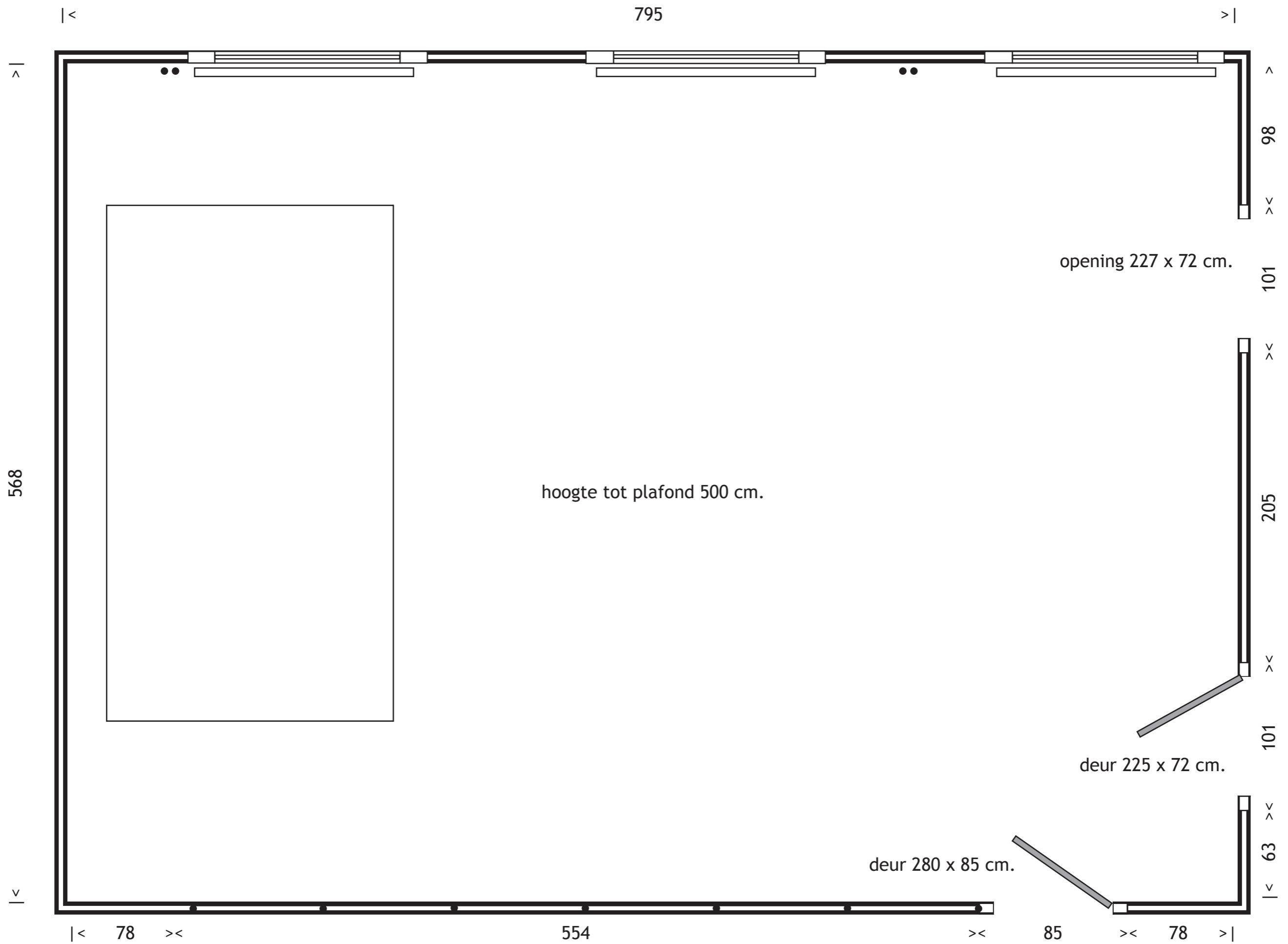
plattegrond podium ocw, begane grond, drievriendenstraat 26 / lokaal 01, 3014 JS rotterdam.
